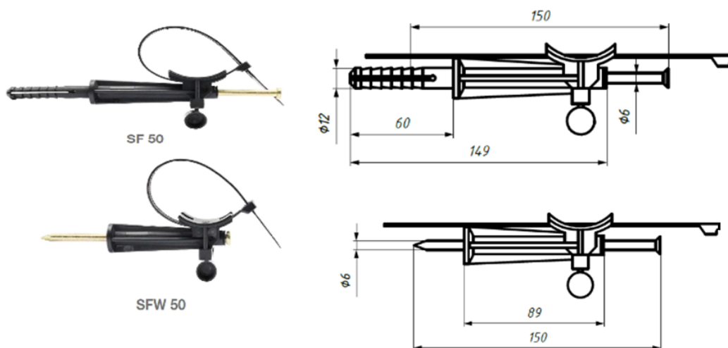
Рис. 1. Внешний вид фасадных креплений SF 50, SFW 50.
