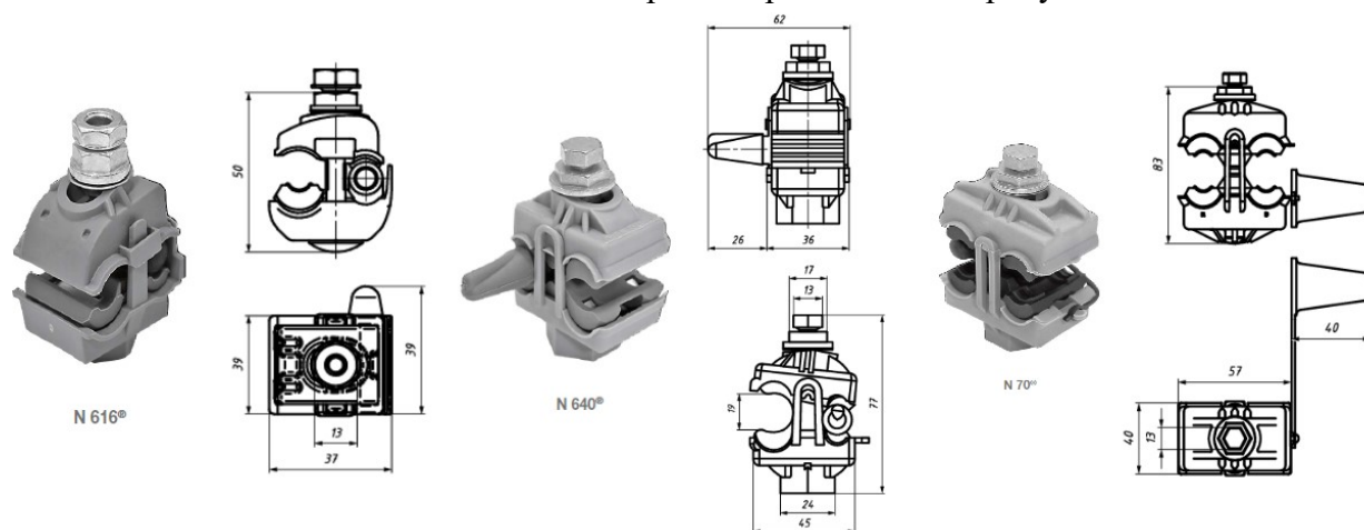
Рис. 1. Внешний вид ответвительных зажимов серии N.
